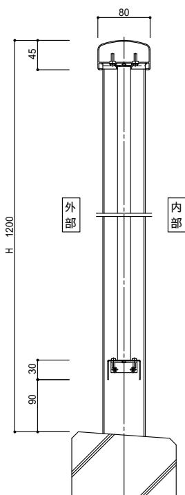
手すり子
