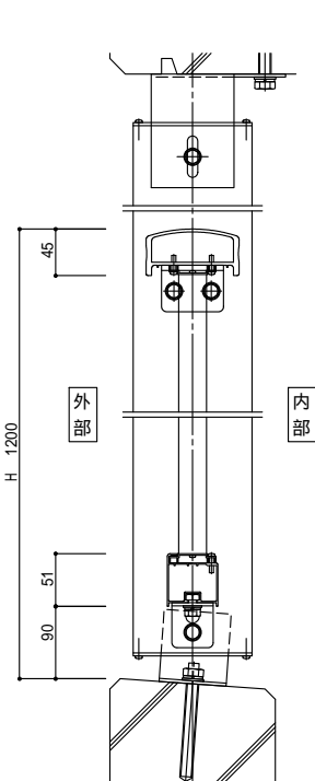
手すり子(方立支持)
