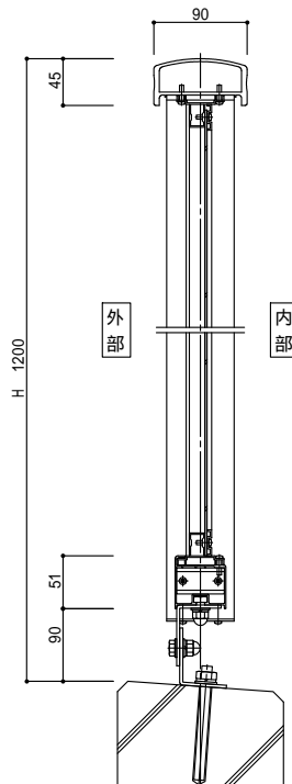
パネル(壁支持)
